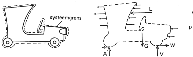
Figuur 1.6. Als de systeemgrens door het contactvlak met een vloeibaar of gasvormig medium loopt moeten ook contactkrachten worden ingevoerd. In het geval van een rijdende auto oefent de rijwind op elk deeloppervlakje een drukkragtje (loodrecht op raakvlak) en een wrijvingskrachtje (in raakvlak) uit. Gesommeerd ontstaat de luchtkracht L . In de figuur is L evenwijdig met het wegdek getekend.
